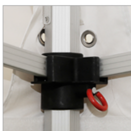
Bague coulissante renforcée
