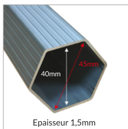
Section des pieds Épaisseur 1,5mm
